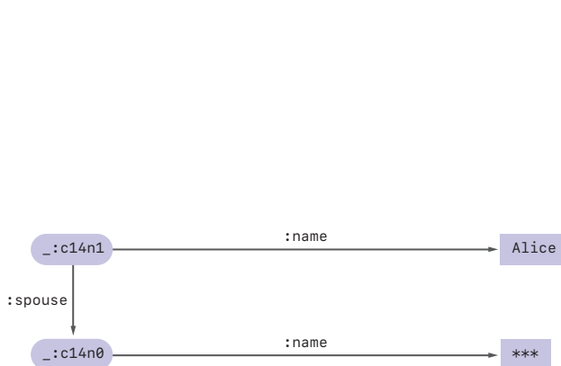
図-10 Bobの名前が隠されたRDFグラフ
