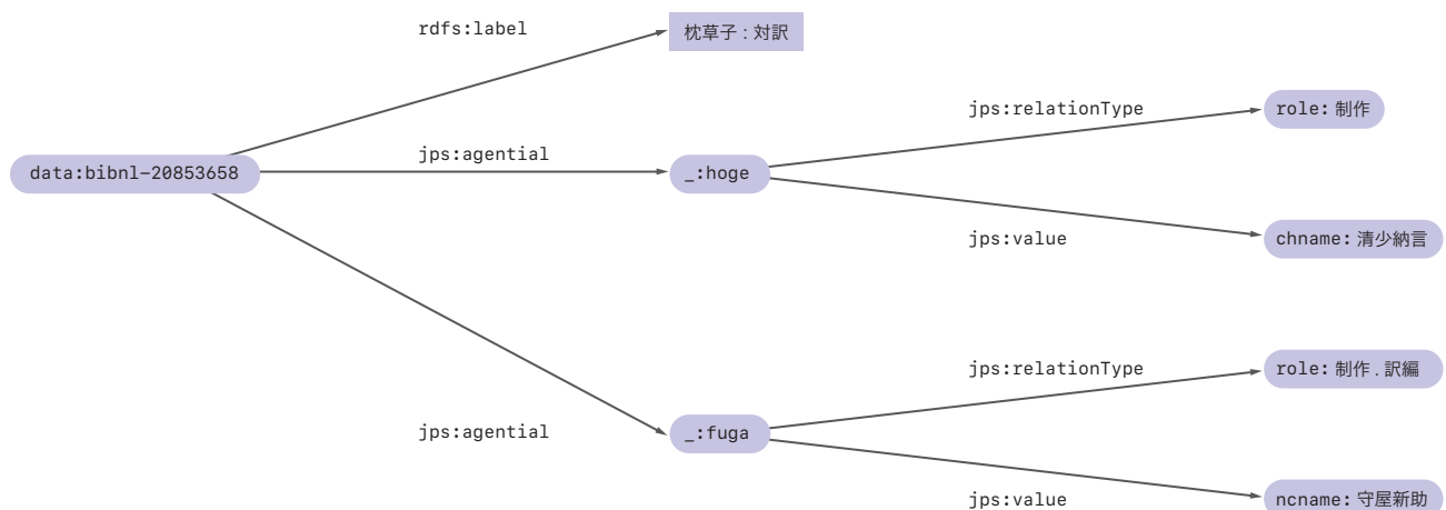
図-3 枕草子に関するRDFグラフのもう1つの例
