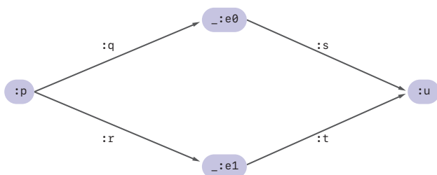
図-6 2つの空白ノードを含むRDFグラフの例
