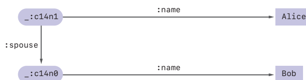
図-9 図-8の正規化後
