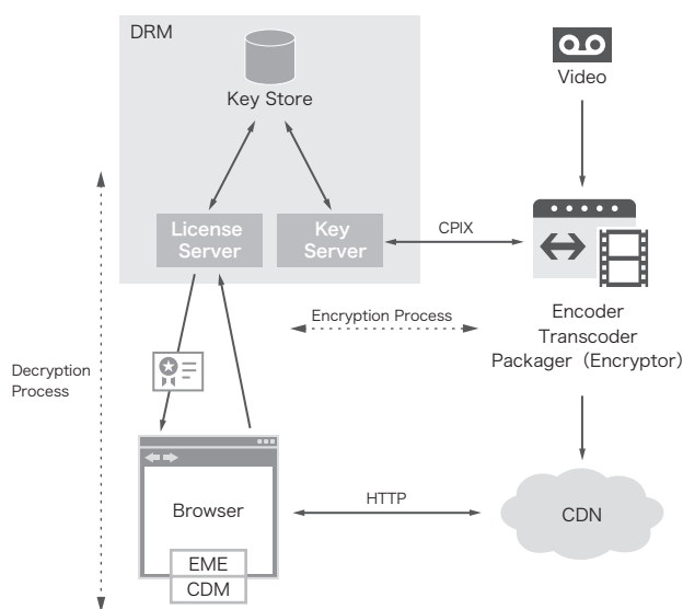
図-1 暗号化と復号の過程
