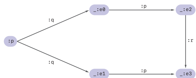
図-7 より複雑なRDFグラフの例
