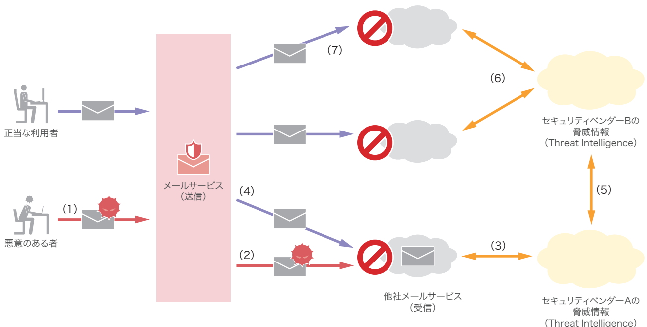
図-1 abuse行為が与えるメールサービスへの悪影響
