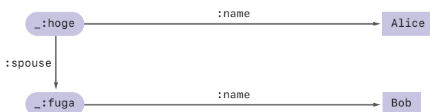
図-8 AliceとBobに関するRDFグラフ
