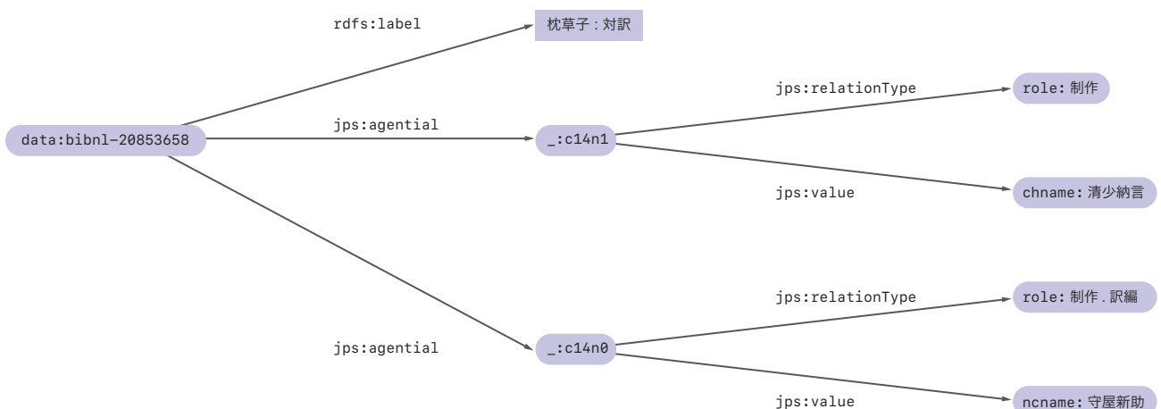
図-4 Canonicalizationを行ったRDFグラフの例
